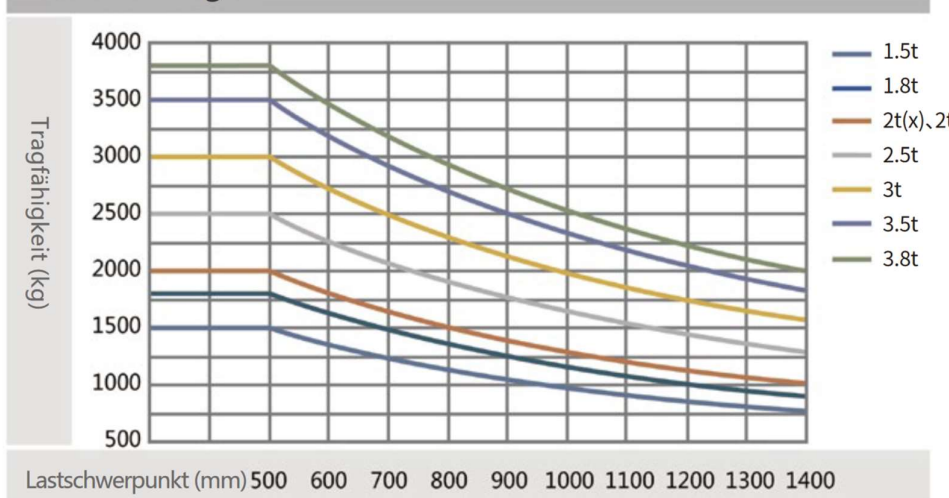
Lastkurven-Diagramm
