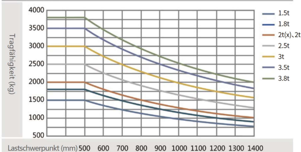
Lastkurven-Diagramm
